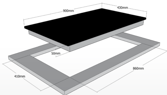
Aufliegender Einbau
