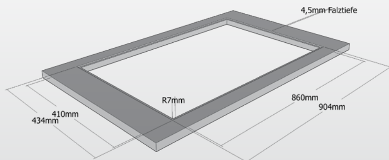
Flächenbündiger Einbau
