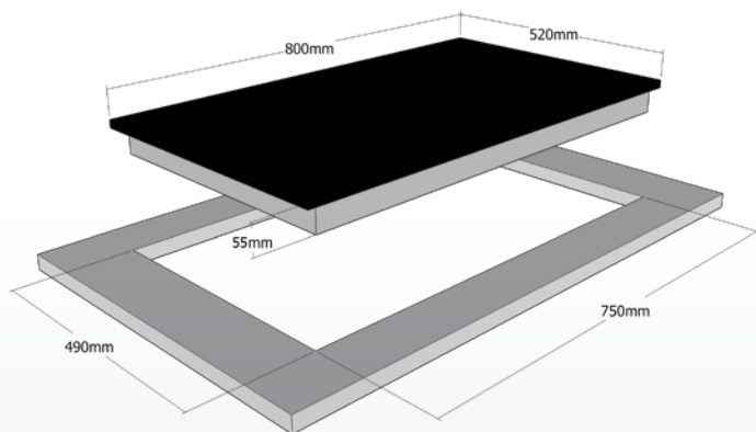
Aufliegender Einbau
