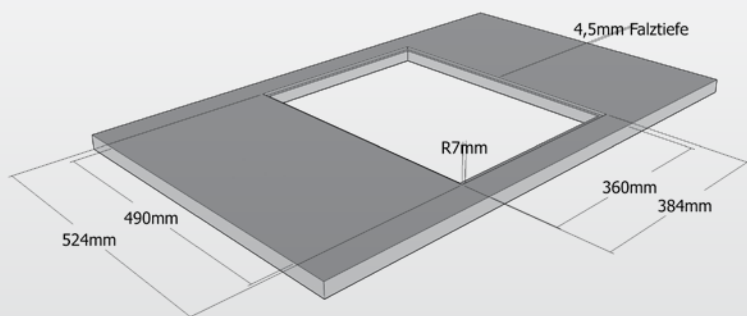
Flächenbündiger Einbau
