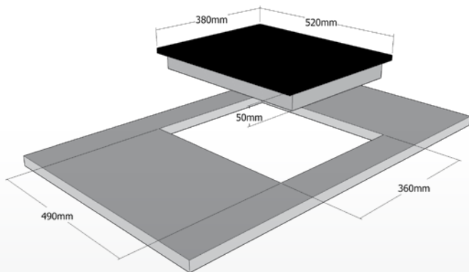
Aufliegender Einbau
