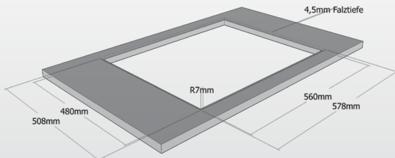
Flächenbündiger Einbau
