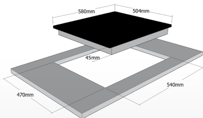
Aufliegender Einbau
