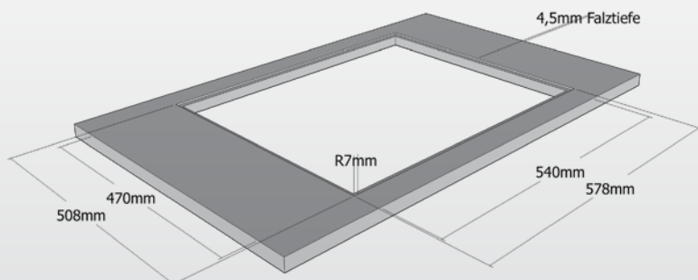
Flächenbündiger Einbau
